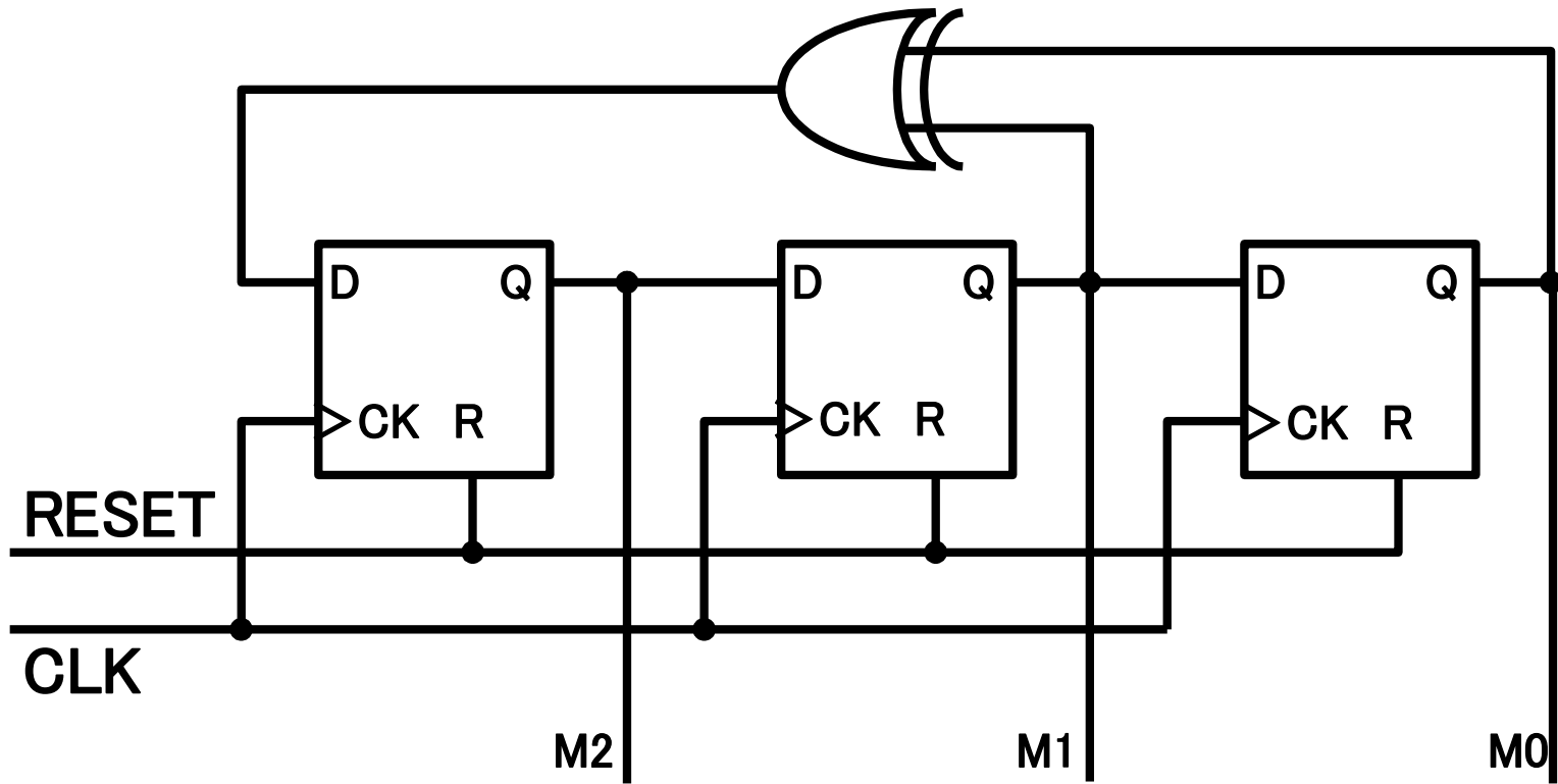
M系列発生器回路
