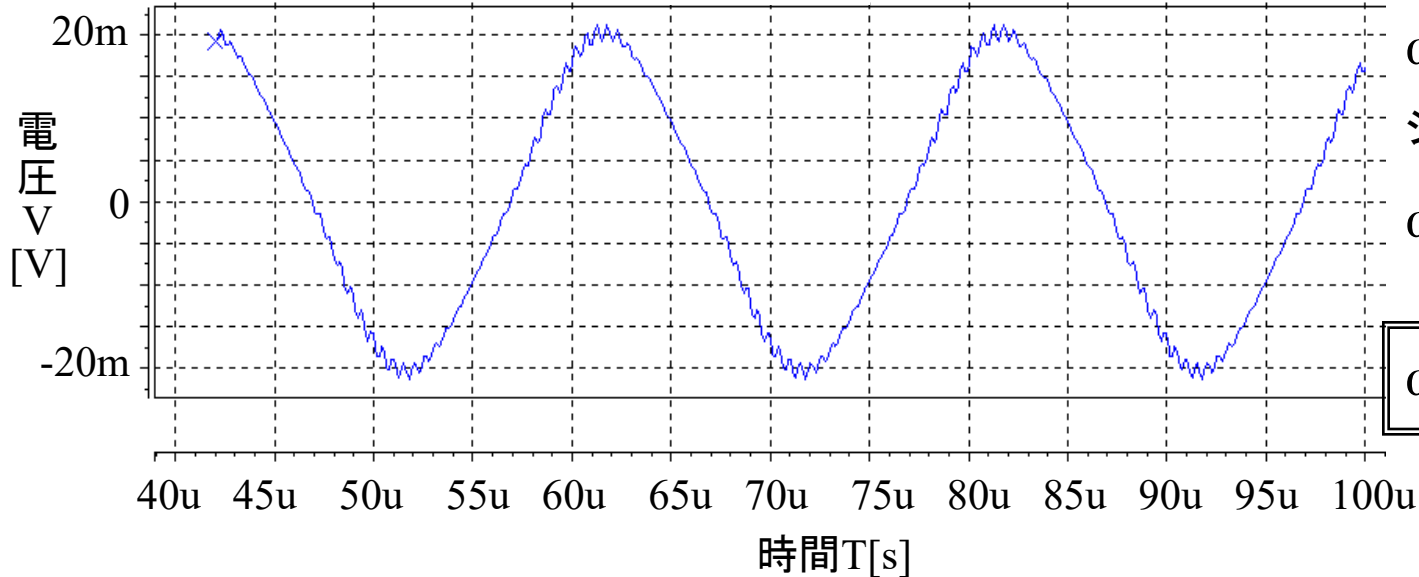
出力波形
