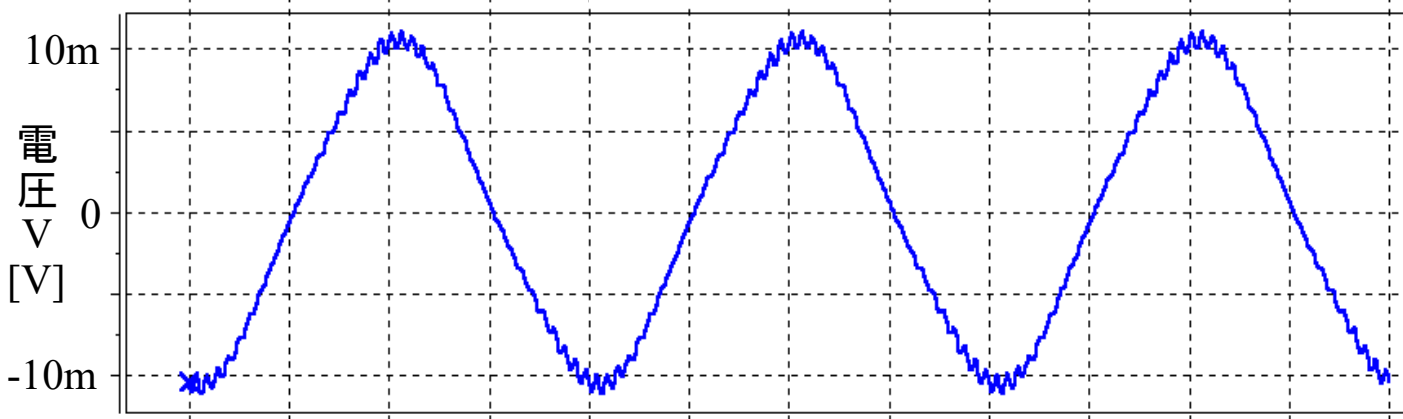
出力波形
