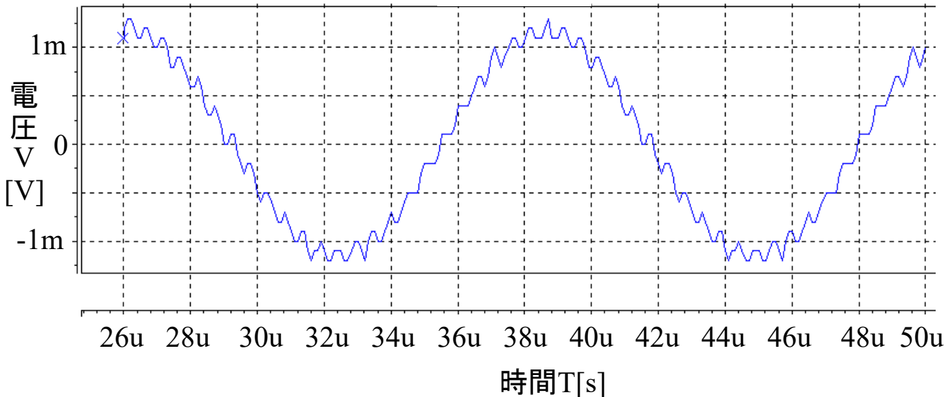
出力波形
