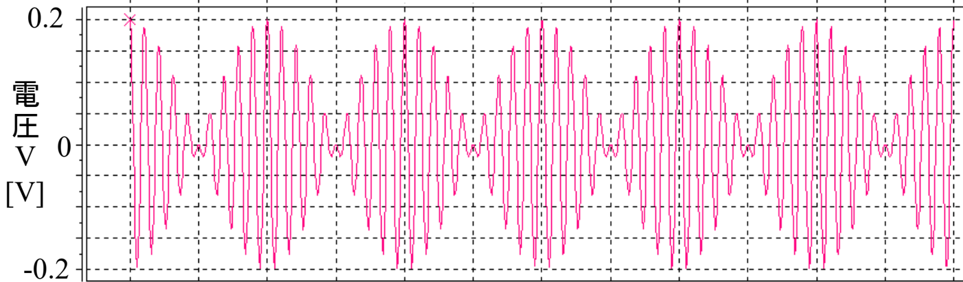
入力波形
