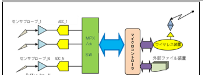
図2. 開発対象伝送系システム図
