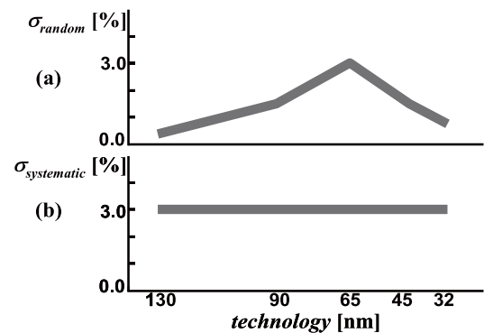
図2 半導体集積回路の「ランダム」ばらつきと「システムティック」ばらつきの推移。S. Natarajan 博士のスライドのメモから。(a)「ランダム」ばらつきは減少傾向。(b)「システムティック」ばらつきは、設計ルール導入により、一定傾向。
