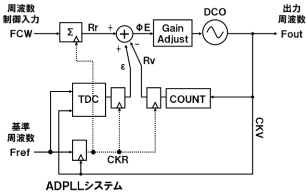
図2 検討した ADPLL 構成
