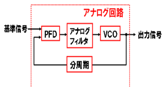
図 1 従来のアナログ PLL 構成
