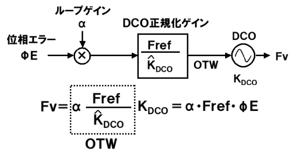
図4: ADPLL ないでの DCO 周辺の構成.
