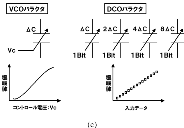
図3. デジタル制御発振回路 (Digitally Controlled Oscillator: DCO) の構成. (a) コア回路. (b) DCO では MOS バラクタを2値で用いる. (c) DCO では容量変化値が離散的 (デジタル).
