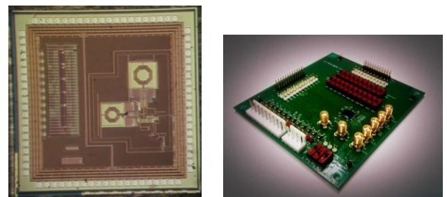
図4: 三洋半導体と開発した完全デジタルPLL-TV チューナLSI を実装した評価基板。0.18 μm CMOS プロセスで設計試作したLSI をワイヤボンディングで評価基板と直接接続し、多数の制御信号ピンやスイッチを基板上に実装することで、より高度な測定評価を可能とした。TV チューナ用完全デジタルPLL LSI の開発は世界初。
